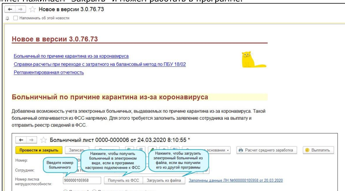
Рис.9 Описание изменений
