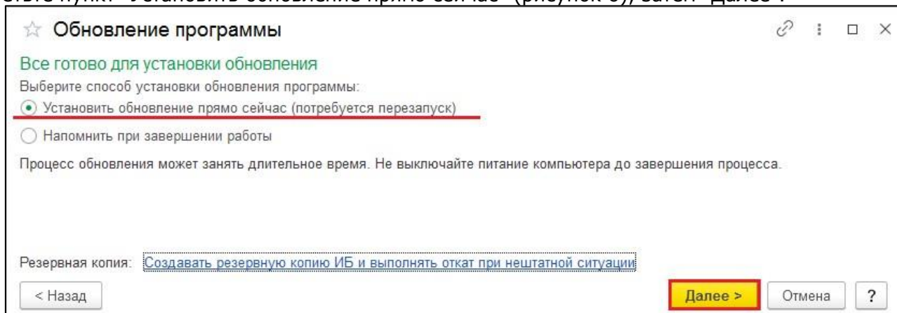
Рис. 6 Запуск автообновления
